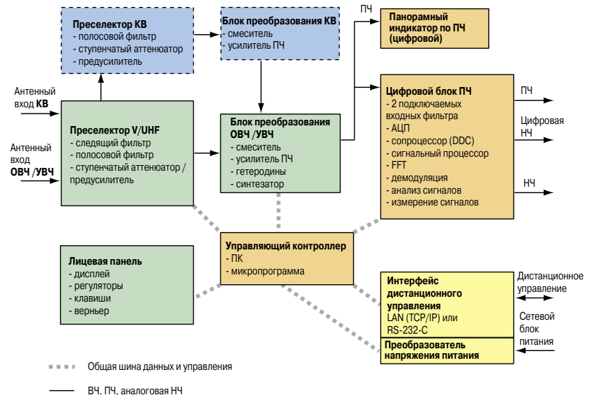
Структурная схема мониторингового приемника ESMB
